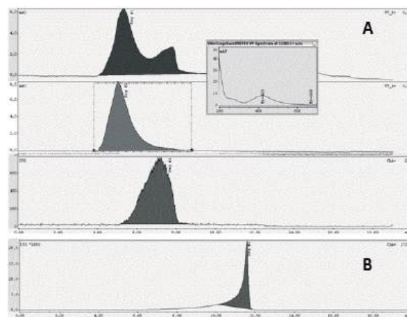
Figura 6A. Perfil de HPLC: 99m Tc-AgNPs-ICG
